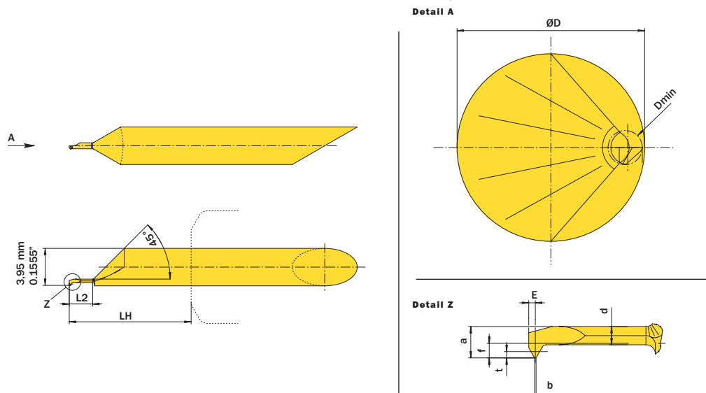
Abbildung zeigt / Drawing shows: A04.M025.01.02.07 MR
